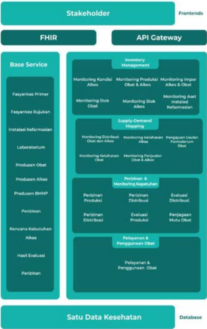
Gambar 22. Arsitektur Ap/Bundel Layanan Farmasi
